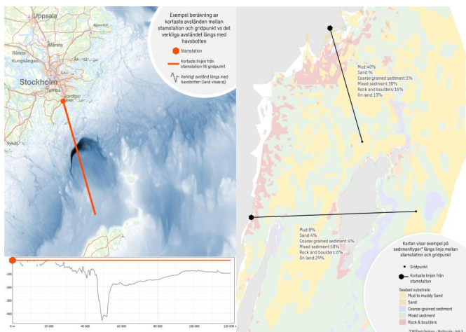
Figur 35. Exempel på batymetrikarta och väg längs botten mot stannätsstation till vänster samt exempel på fördelning av ytsediment längs botten på väg mot stannätsstation till höger.
