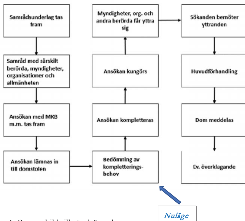
Figur 1. Processbild tillståndsärenden.
