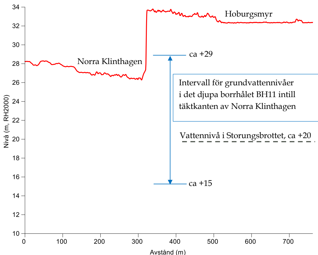
Figur 7. Profil över marknivå mellan Norra Klinthagen och Hoburgsmyr.
