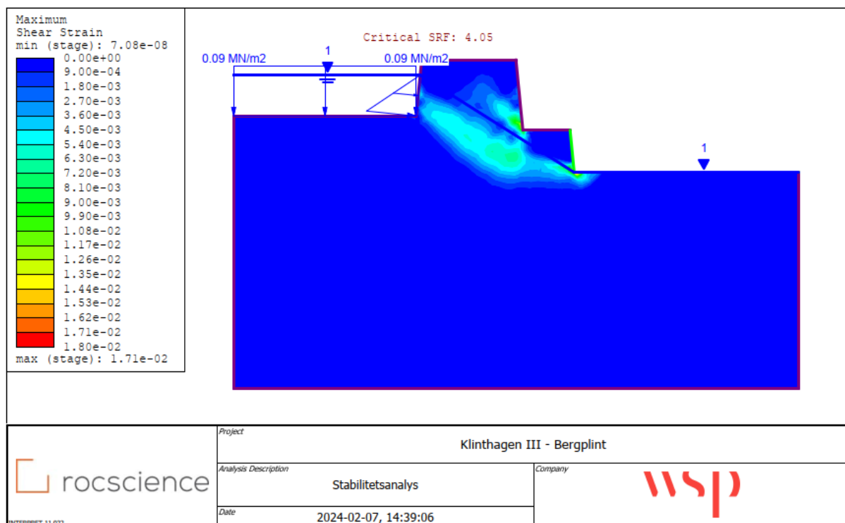
Figur A-7. Maximal töjning vid brott under reduktionsanalys.
