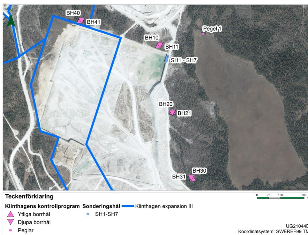
Figur 28. Läge över borrhålspar som ingår i Klinthagens kontrollprogram och pegel vid slukhål i Hoburgsmyr, samt läge för sonderingshål utanför tätkant i nordost.
