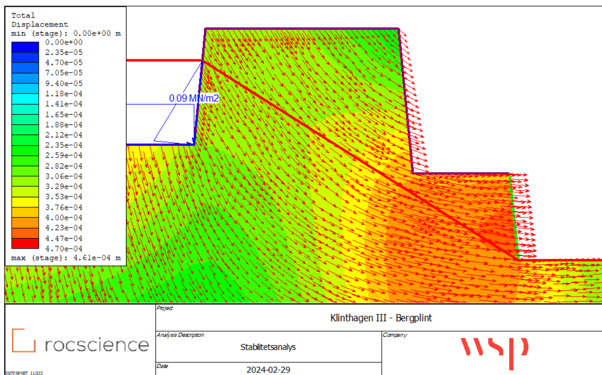
Figur 4-1. Beräknad deformation under belastning. Röd linje representerar yt- och grundvattennivån. Pilarna visar rörelseriktningen.
