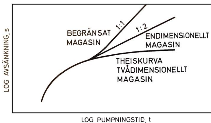
Figur 25. Avsänkingskurvas form vid olika magasinstyper (Carlsson & Gustafson, 1997).
