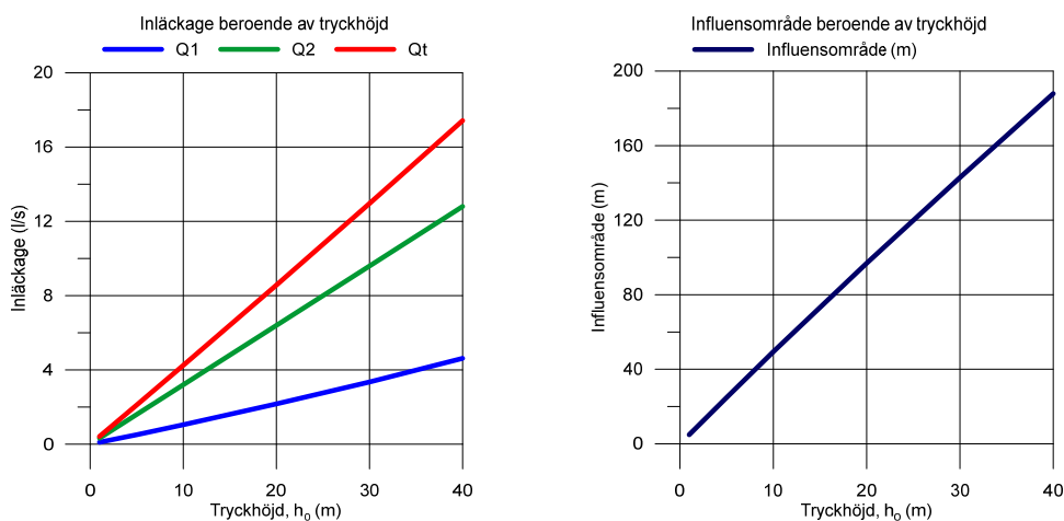
Figur 44 - utgått. Känslighetsanalys vid variabelt värde på omgivande grundvattennivå. Q1 är det horisontella flödet in i tätten och Q2 är det vertikala flödet genom botten av tätten, enligt beräkningsmodell som redovisas i Figur 34.
