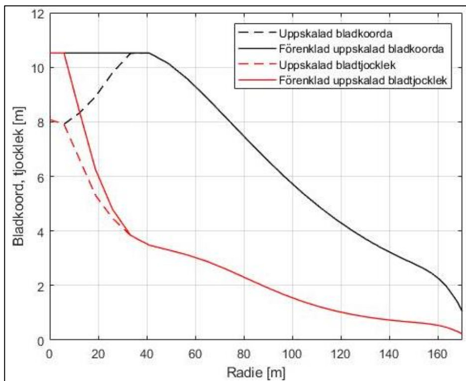
Figur 3: Bladkoorda och bladtjocklek.
