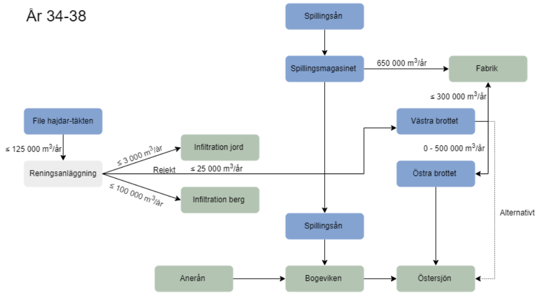
Figur 5. Flödesschema över den ansöka verksamheten år 34–38.
