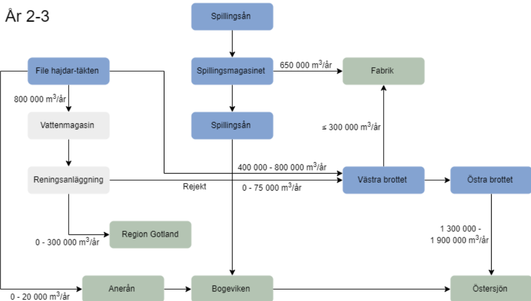
Figur 2. Flödesschema över den ansökta verksamheten år 2–3.
