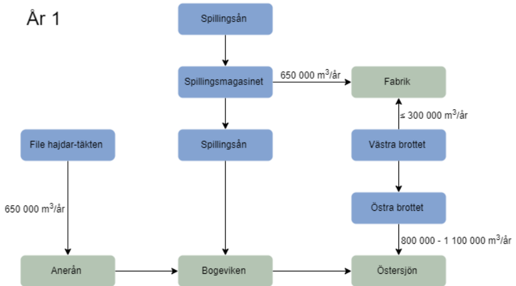
Figur 1. Flödesschema över den ansökta verksamheten år 1.
