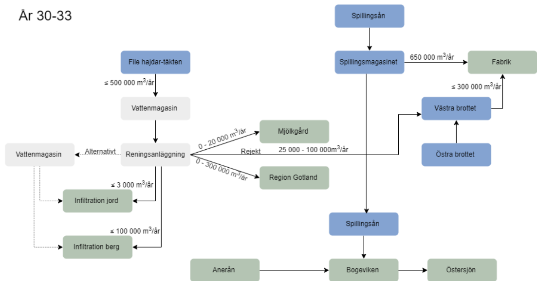
Figur 4. Flödesschema över den ansöka verksamheten år 30–33.
