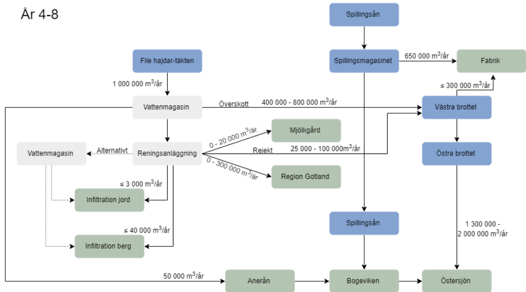
Figur 3. Flödesschema över den ansöka verksamheten år 4–8.
