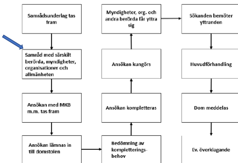
Figur 1. Processbild tillståndsärenden.
